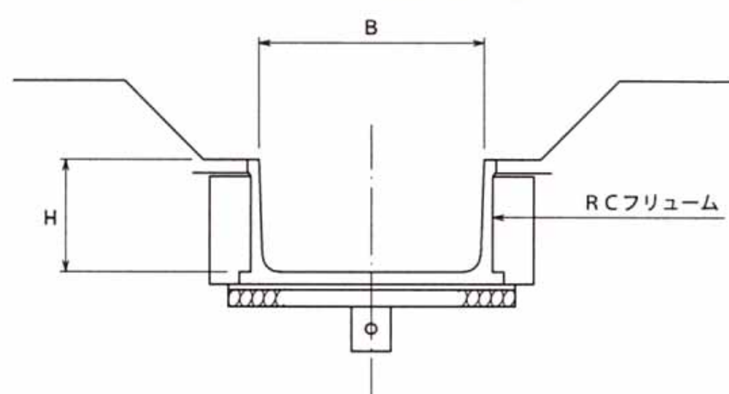
I、II、IV型開渠工
