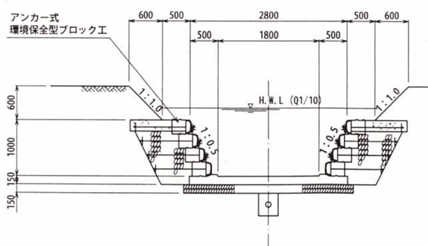
III型開渠工(環境保全型)
