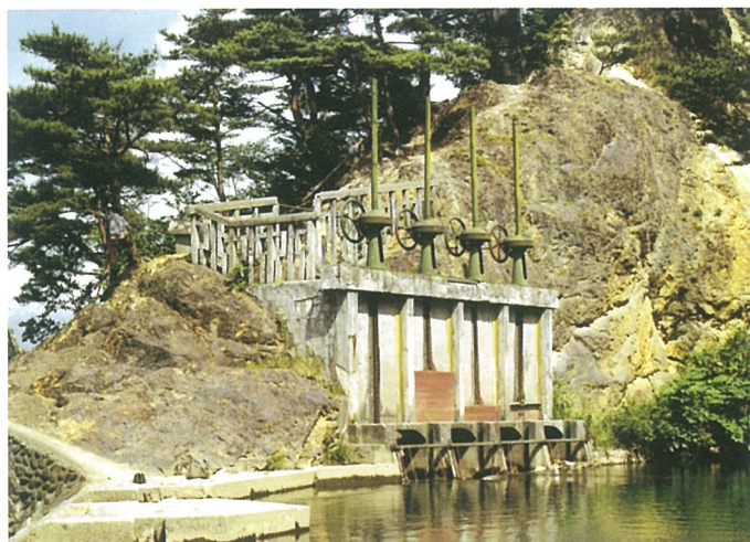
旧鹿妻穴堰頭首工
